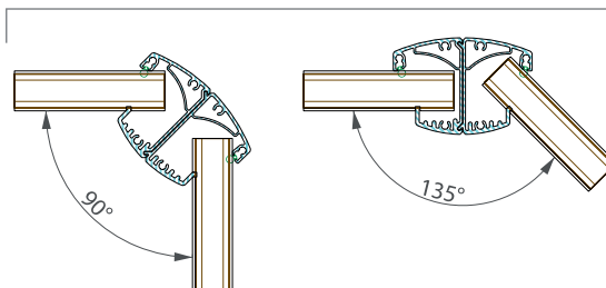
rohový sloupek (90° - 179°)
