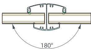
napojovací sloupek
