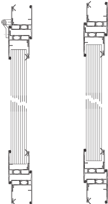
svislý řez
